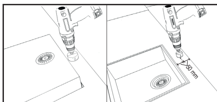
Afb. 6a - 57 mm kraangat boren (onderzijde)
